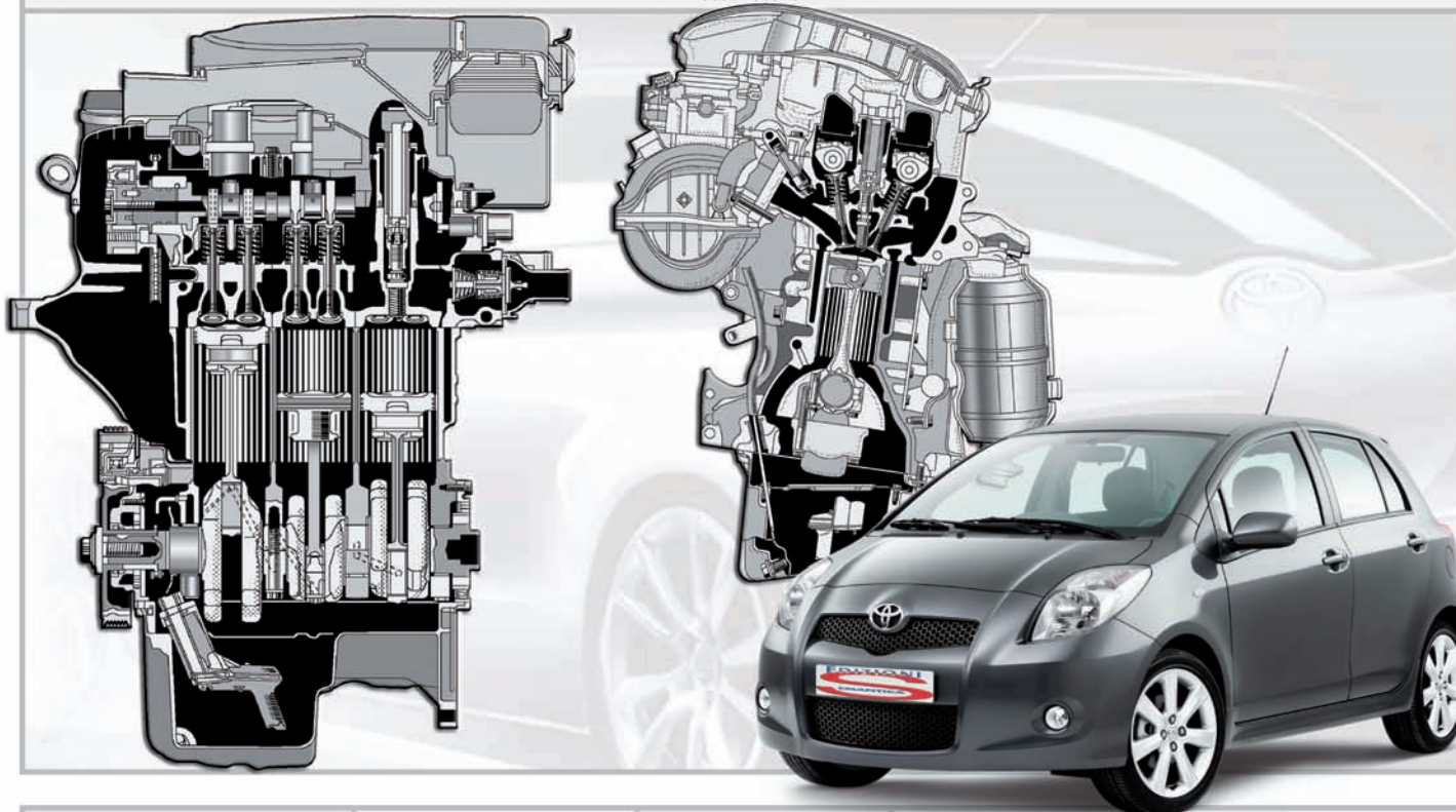
Viste motore
